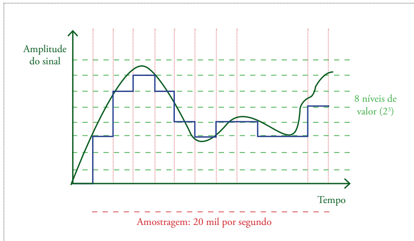
Figura 5 – Amostragem de sinal analógico (2bits)
