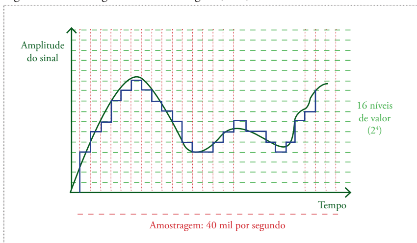
Figura 6 – Amostragem de sinal analógico (8bits)
