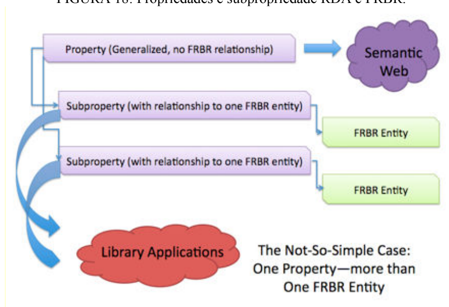
FIGURA 18: Propriedades e subpropriedade RDA e FRBR.
