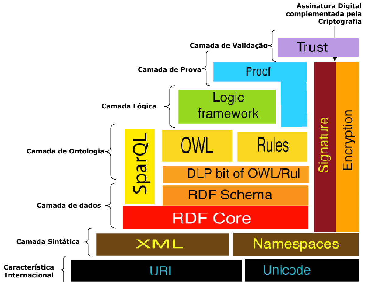
FIGURA 3: Arquitetura da Web Semântica comentada pelo autor.
